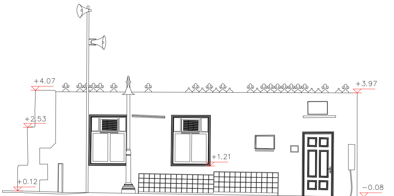
الواجهة الشماليه A 05 Elevation no . 1
